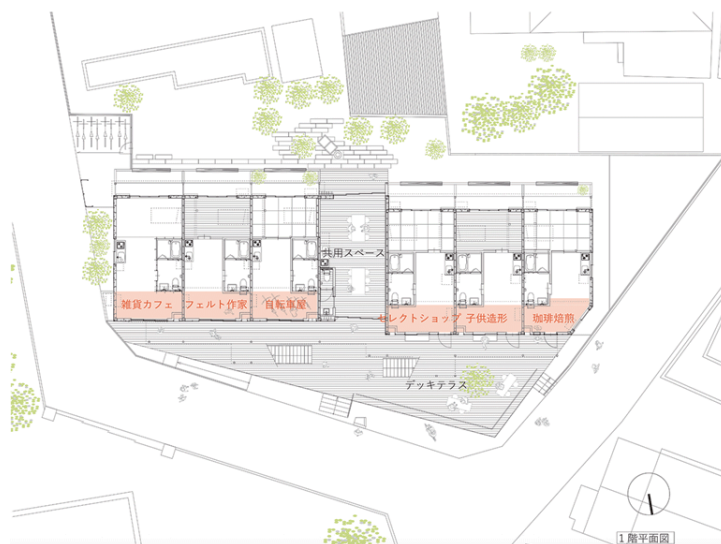
1階平面図
