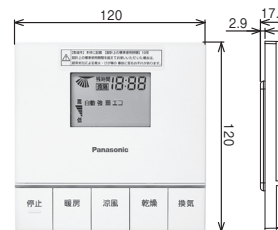
リモコン外形図(ABD-4121ACSK-L用)
