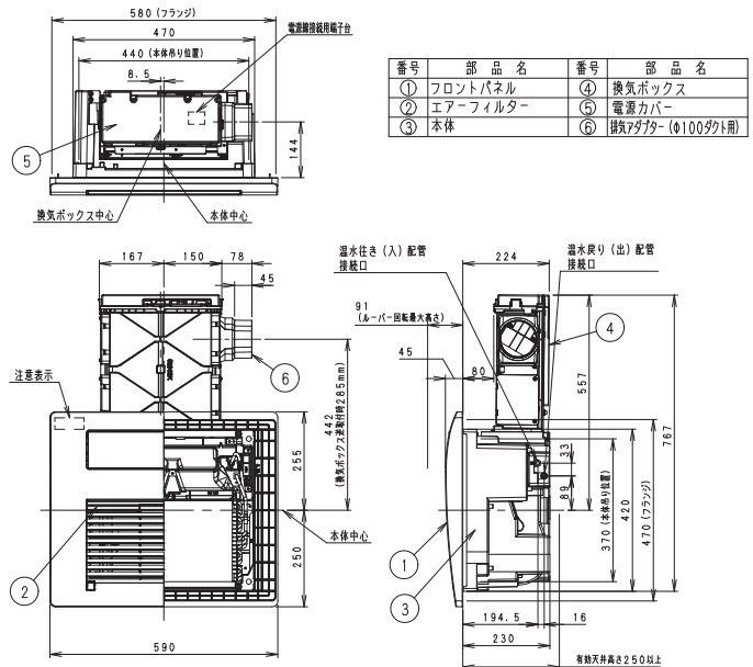
寸法図 単位:mm
