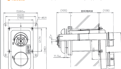
TFW-100A1シリーズ(一体型) TFW-80C2シリーズ(一体型)
