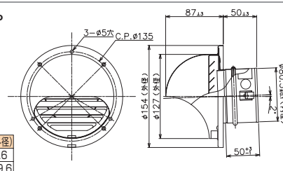
TZ-FBW80NKP/100NKP
