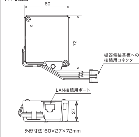
本体寸法図
