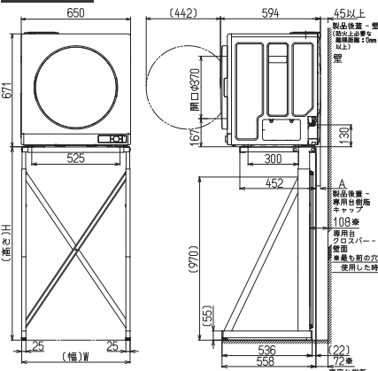
専用台:DS-54HSF
