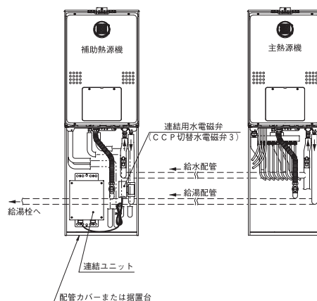
■連結ユニットを配管カバー内に設置する場合
