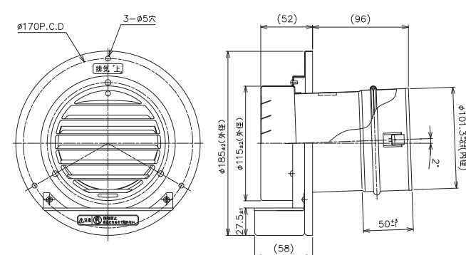
寸法図 TFB-100(D)&lt;排気トップ&gt;
