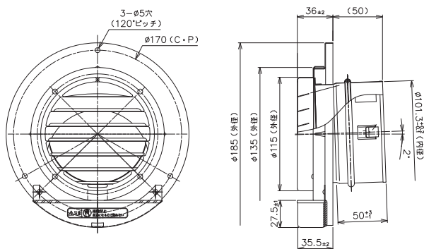
寸法図 TZ-FBW100NKP(D)ストレート
