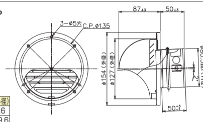
寸法図 TZ-FBW80NKP
