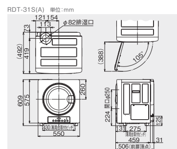
スタンダード3kgタイプ RDT-31S(A)
