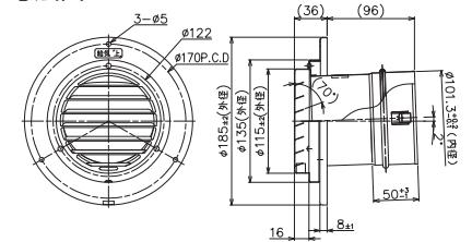
寸法図 TFB-100B(分離型) (排気トップ)
