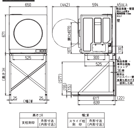
専用台:DS-80MSF
