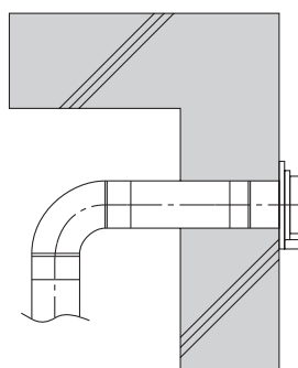
〈外壁貫通の場合〉
