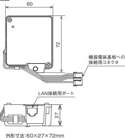
本体寸法図
