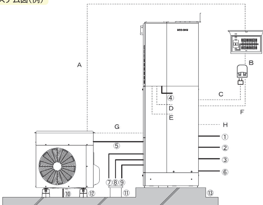
一体タイプシステム図(例)
