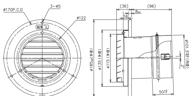
寸法図 TFB-100(D)&lt;給気トップ&gt;
