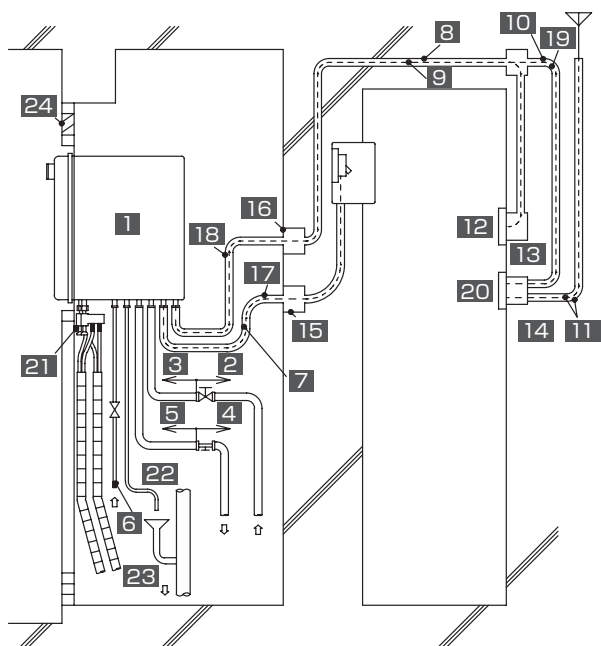
排気延長(例)
