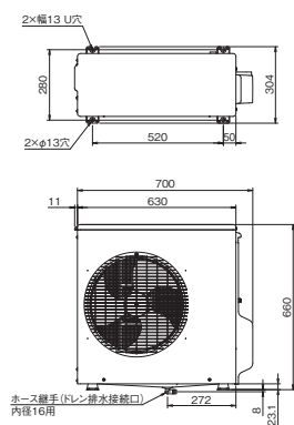
ヒートポンプユニット
