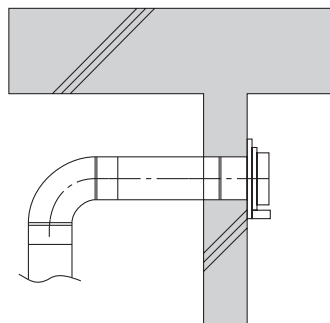
〈PS・梁貫通の場合〉
