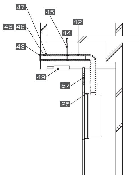
排気延長(例)
