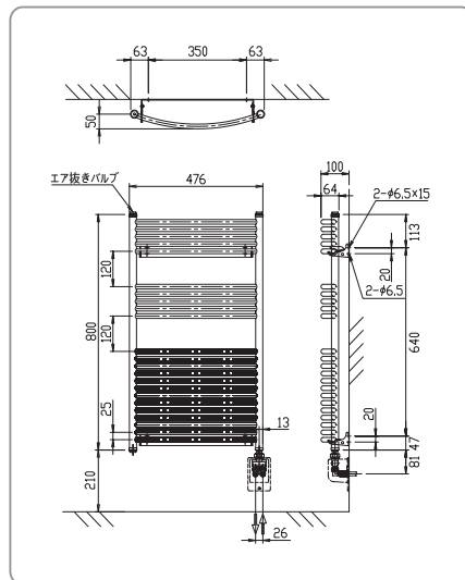
寸法図(ZIR-0403AWN-0804)
