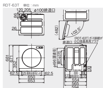
デラックス6kgタイプ (上部操作モデル) RDT-63T
