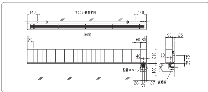
寸法図(ZIR-1303AWN-0216)
