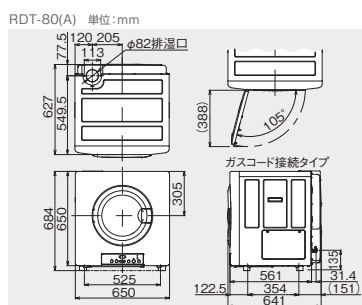
スタンダード8kgタイプ RDT-80(A)
