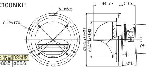
寸法図 TZ-FBC100NKP
