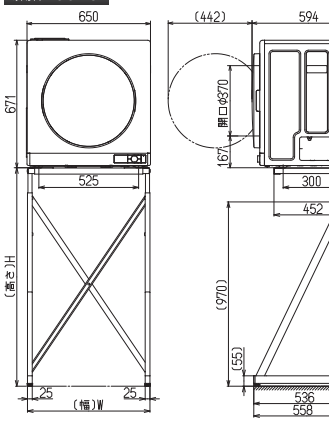
専用台:DS-54HSF
