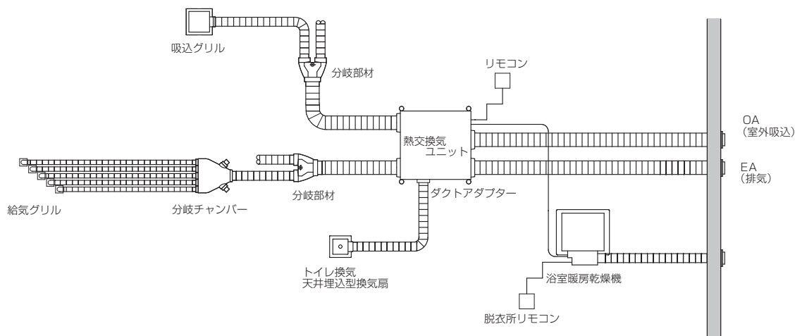
■AIR TESシステム構成例平面図
