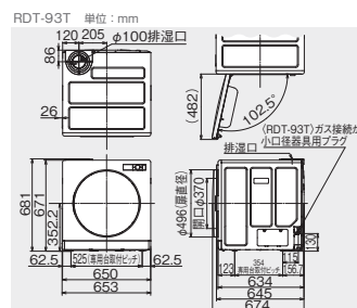
デラックス9kgタイプ (上部操作モデル) RDT-93T
