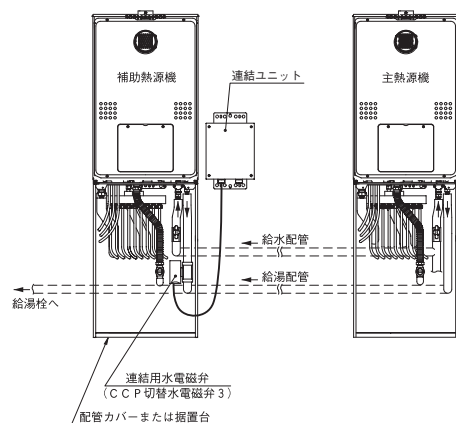
■連結ユニットを配管カバーの外に設置する場合
