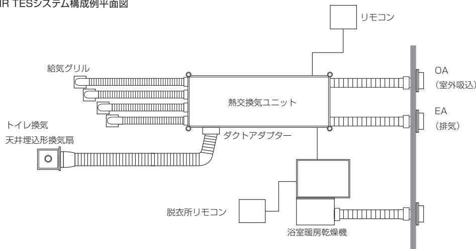
■AIR TESシステム構成例平面図
