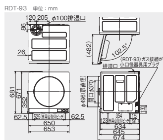
デラックス9kgタイプ RDT-93
