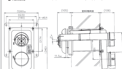
寸法図 TFW-100A1シリーズ(一体型)
