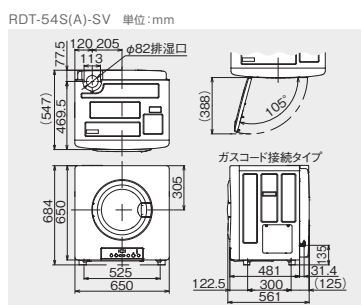
スタンダード5kgタイプ RDT-54S(A)-SV
