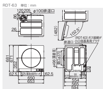
デラックス6kgタイプ RDT-63
