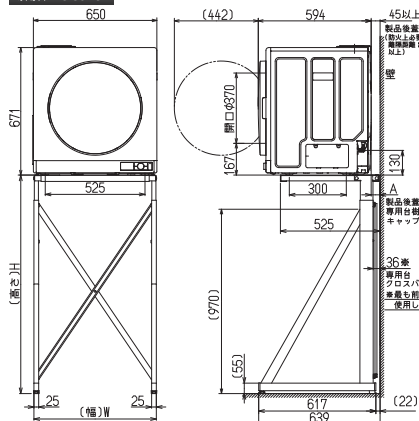
専用台:DS-80HSF
