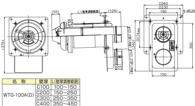
寸法図 WTG-100A(D)Cシリーズ(一体型)
