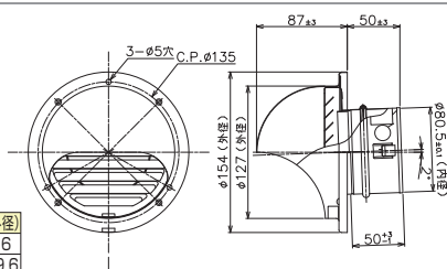
寸法図 TZ-FBC80NKP
