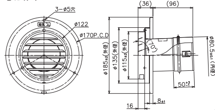
寸法図 TFB-80B (排気トップ)
