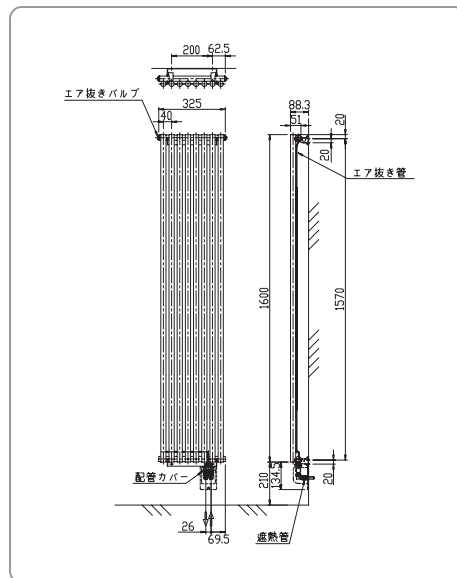
寸法図(ZIR-0703AWN-1603)
