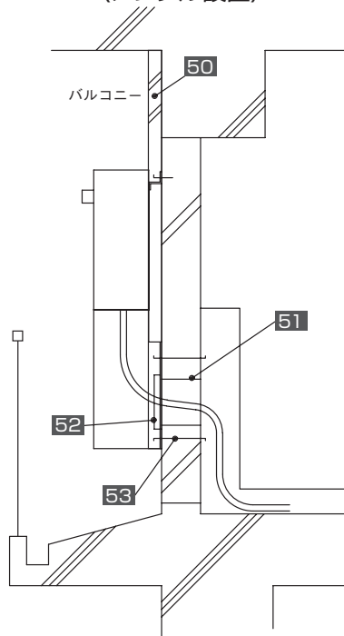
〈アングル設置〉
